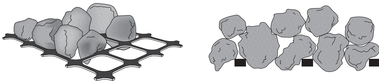
Figur V2.4 Geonett. Kraftene overføres gjennom mekanisk forking av gruskornene. Tverrribbene gir forankring i omliggende masser.
