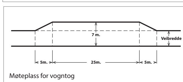
Figur 3.10 Snu- og møteplasser, veiklasse 3.
